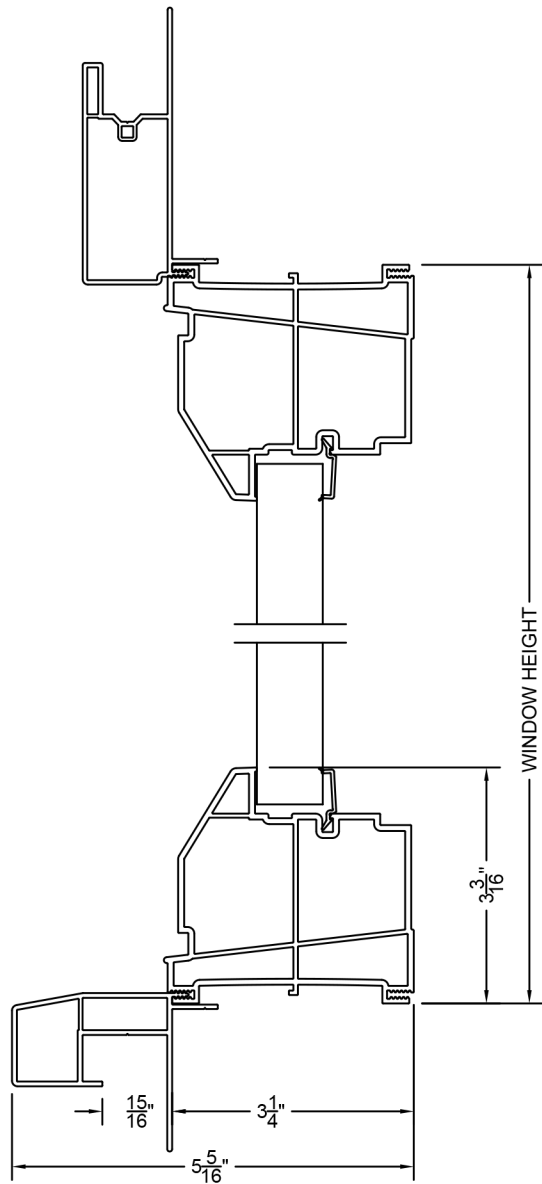
SECTION A-A SCALE: 1:1
